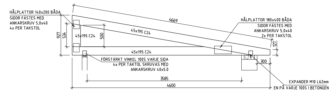
TAKSTOL T2 150 TAKSTOL T3 LIKA HÖJD MED LÄNGD I PLAN. TAKÅSAR MÄTTAS PÅ PLATS MED TAKFALL SOM FÖLJER T1.
