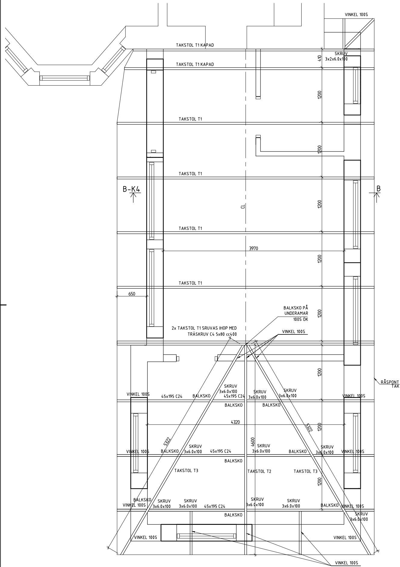
TAKSTOLSPLAN 150
